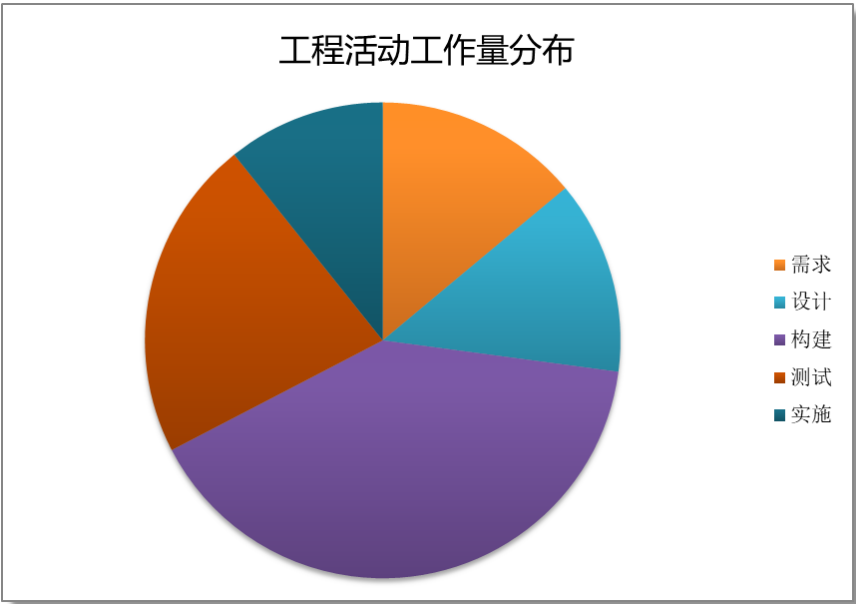
图 3.6 工作量分布
