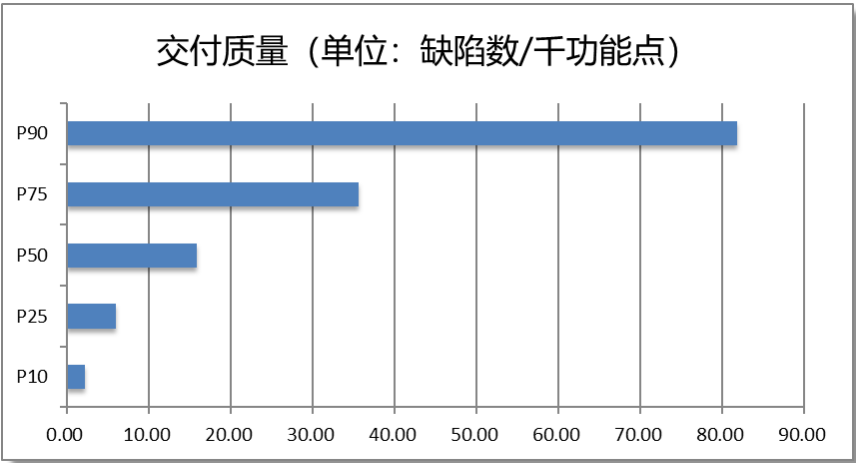
图 3.5 交付质量
