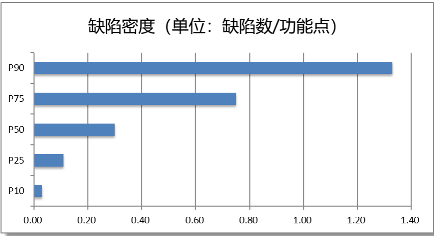
图 3.4 缺陷密度
