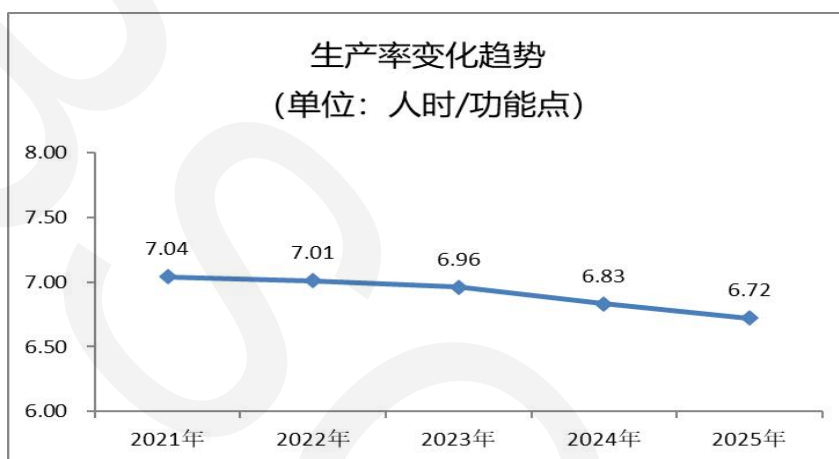
图 6.1 全行业软件开发生产率变化趋势
