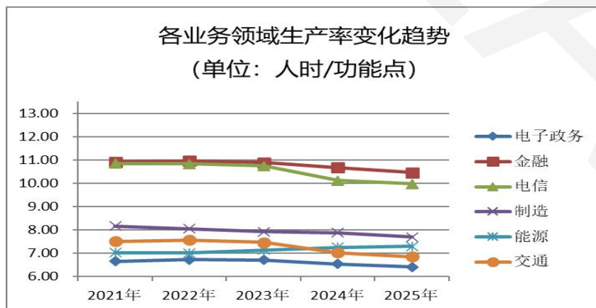
图 6.2 各业务领域软件开发生产率变化趋势
