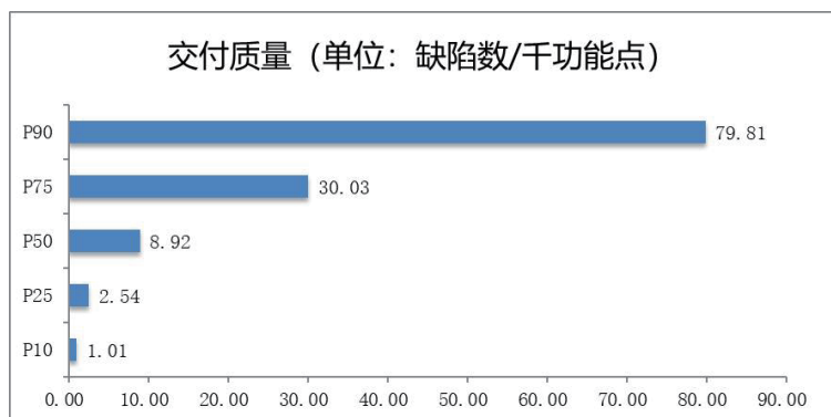
图 4.5 交付质量
