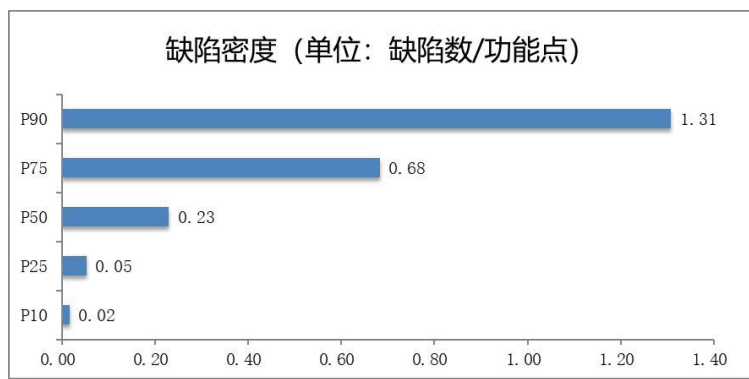
图 4.4 缺陷密度
