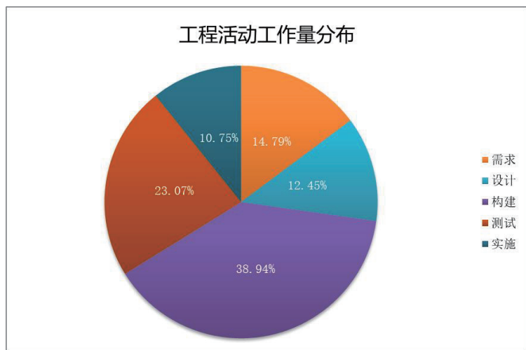
图 4.6 工作量分布
